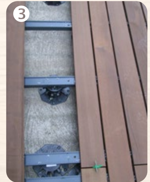
TERRASSEN AUFBAU Der Unterbau ist für eine dauerhafte Terrasse ausschlaggebend.
